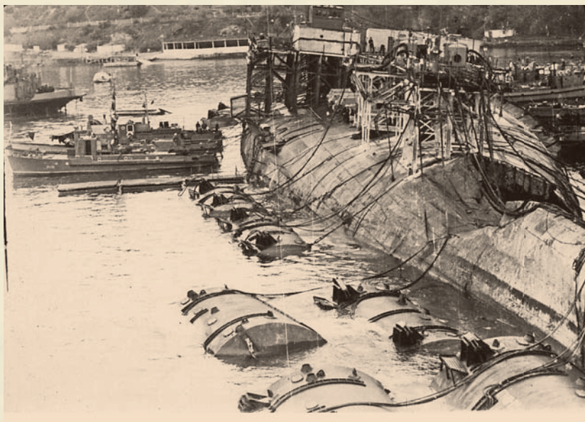
ПОДЪЕМ ЛИНКОРА «НОВОРОССИЙСК»
