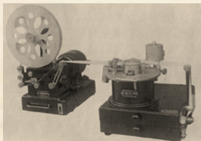
ОНДУЛЯТОР ОТ РАЦИИ «45 ПК-1» (СПРАВА), ЗАПИСЫВАВШИЙ НА ДВИЖУЩЕЙСЯ БУМАЖНОЙ ЛЕНТЕ ЗНАКИ КОДА МОРЗЕ В ВИДЕ ЗИГЗАГООБРАЗНОЙ ЛИНИИ, ПРИМЕНЯЛСЯ И В НЕКОТОРЫХ ПИЩУЩИХ ТЕЛЕГРАФНЫХ АППАРАТАХ
