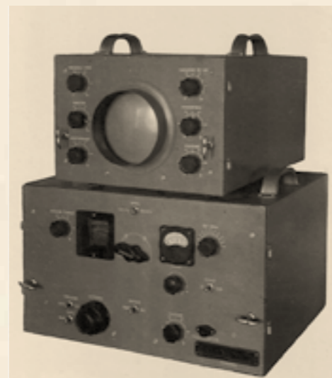
ПРИЕМНИК С ВЫПРЯМИТЕЛЕМ И СТАБИЛИЗАТОРОМ РАДИОСТАНЦИИ «СВ»
